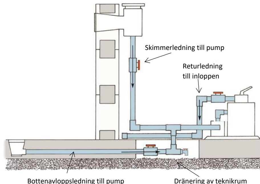
Schematiska ritningar över rördragningen runt poolen.
